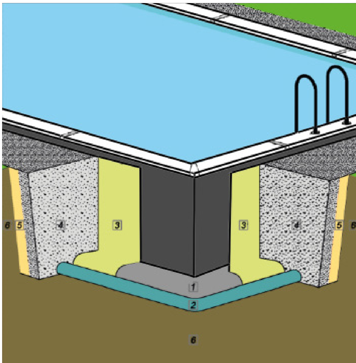
Schéma d'installation d'une structure partiellement ou totalement enterrée
